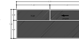
V4 3 PIEZAS ESC: 1:25 CANCERIA A BASE DE PERFIL DE ALUMINIO DE 3" EN COLOR NATURAL Y CRISTAL TINTEX VERDE DE 6 MM DE ESPESOR. VENTILA CORREDIZA, INCLUYE MOSQUITERO.
