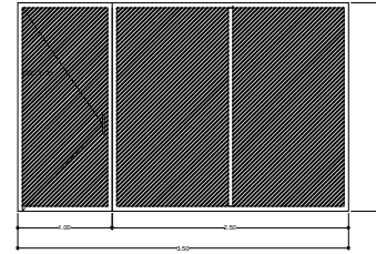
C4 2 PIEZAS CANCERIA A BASE DE PERFIL DE ALUMINIO DE 3" Y PUERTA EN COLOR NATURAL Y CRISTAL TINTEX VERDE DE 6 MM DE ESPESOR.
