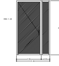
C3 2 PIEZAS ESC: 1:25 CANCERIA A BASE DE PERFIL DE ALUMINIO DE 3" CON PUERTA ABATIBLE EN COLOR NATURAL Y CRISTAL TINTEX VERDE DE 6 MM DE ESPESOR.
