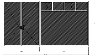
C1 1 PIEZA ESC: 1:25 CANCERIA Y PUERTA ABATIBLE DE DOS HOJAS A BASE DE PERFIL DE ALUMINIO DE 3" EN COLOR NATURAL Y CRISTAL TINTEX VERDE DE 6 MM DE ESPESOR CON PANTALLA A BASE DE PIELICULA ACHISABLE ACABADO ESMERILADO DE 10 CM DE ANCHO. VENTILA CORREDIZA, INCLUYE MOSQUITERO.
