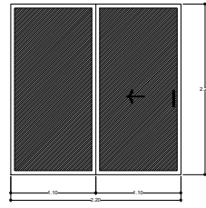
C2 2 PIEZAS ESC: 1:25 1 PTA. HOGA DERECHA Y OTRA A LA IZQUIERDA. CANCELERIA A BASE DE PERFIL DE ALUMINIO DE 3" CON PUERTA CORREDIZA, EN COLOR NATURAL Y CRISTAL TINTEX VERDE DE 6 MM DE ESPESOR, ACABADO ESMERILADO.
