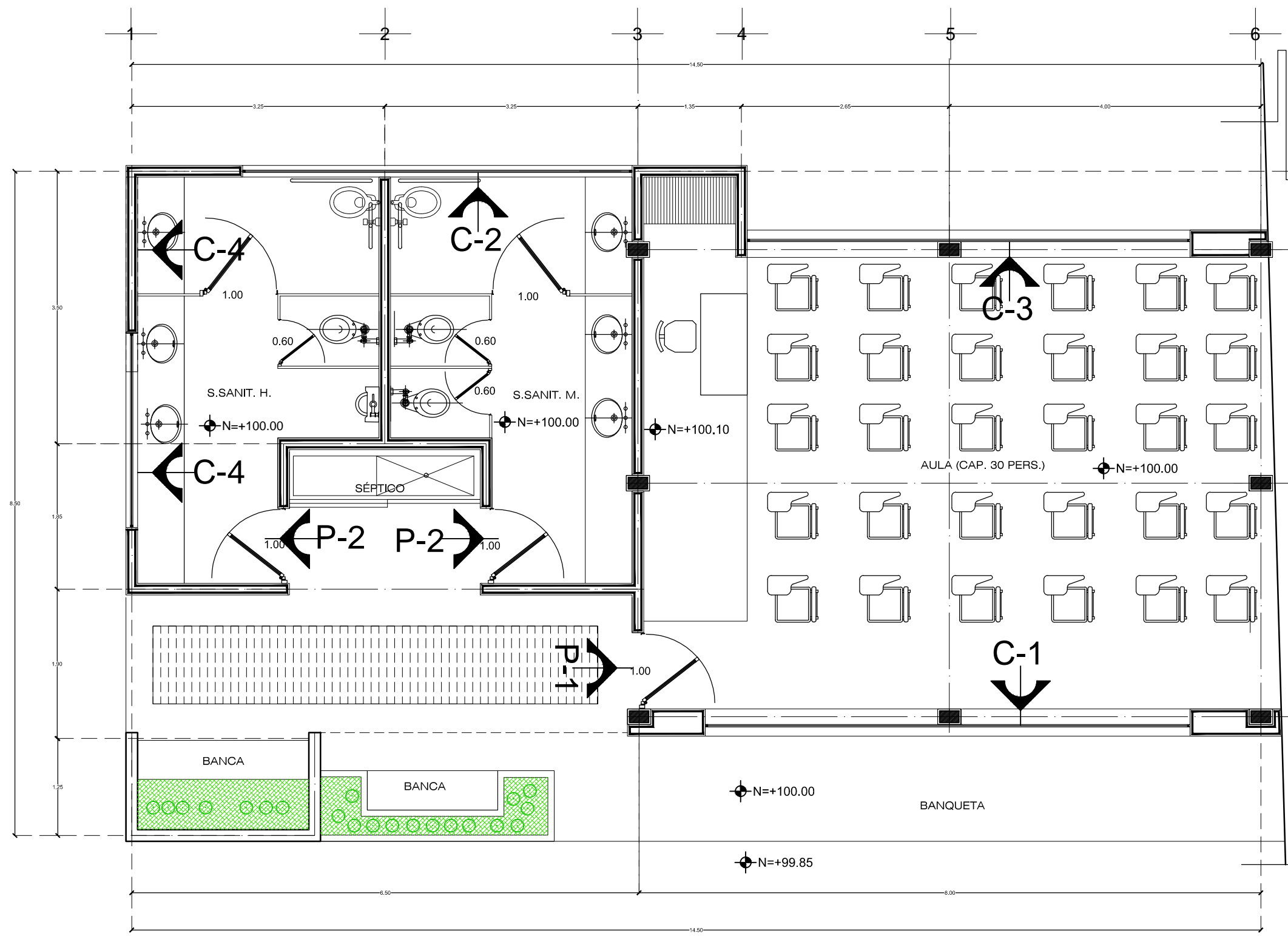
LOCALIZACION DE CANCELERIAS ESCALA 1:25 SUPERFICIE CONSTRUIDA 101.00M2
