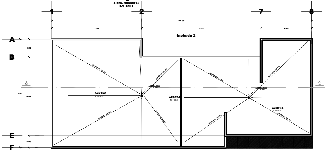
PLANTA DE AZOTEA E S C A L A 1 : 50
