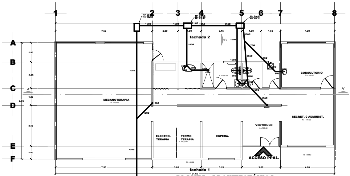
PLANTA ARQUITECTÓNICA E S C A L A 1 : 50 SUP. CONSTRUIDA 185.75M2
