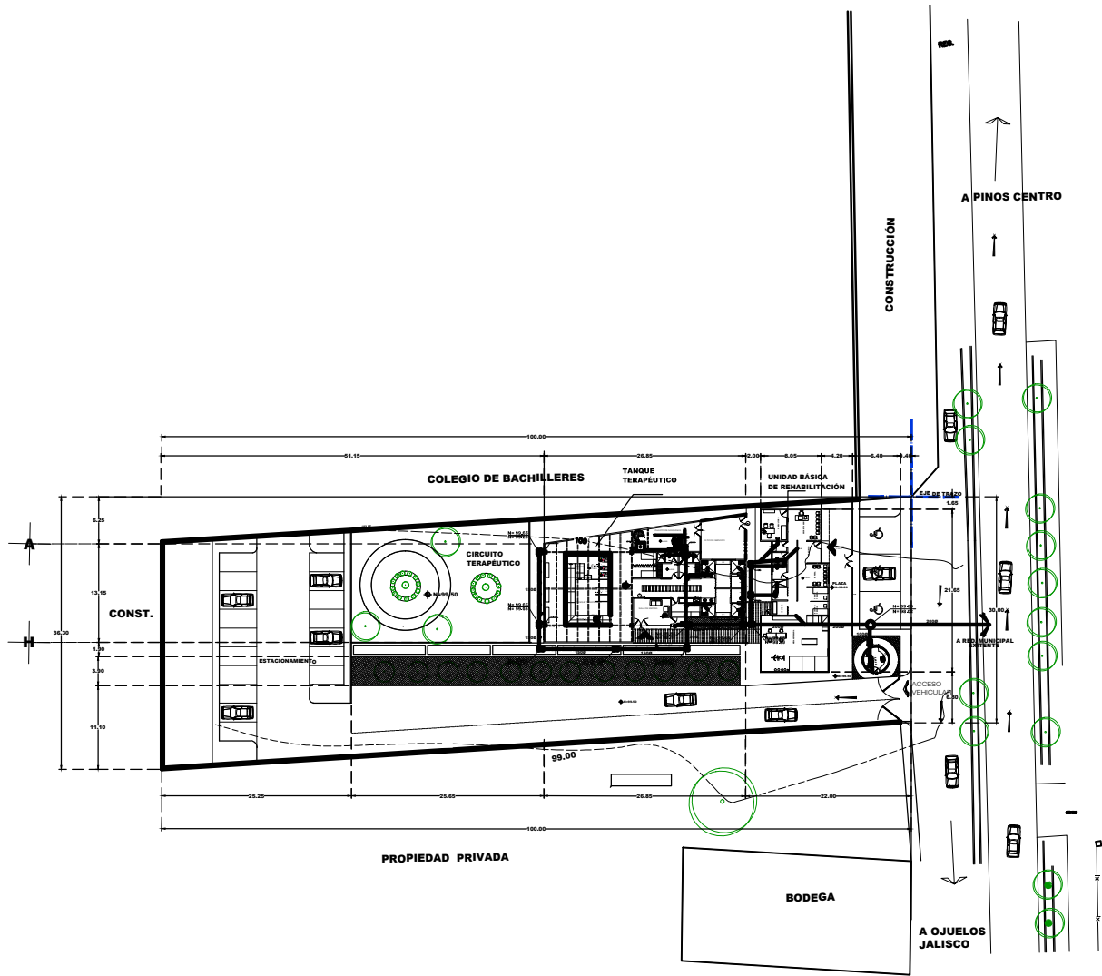
PLANTA DE CONJUNTO ESCALA 1 : 250
